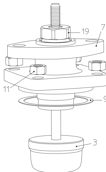
Рис. 24: BR 440 / 445 DN15-100
