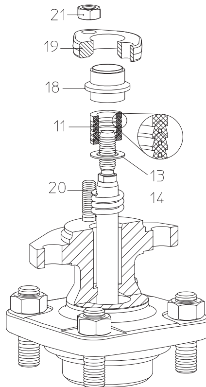
Рис. 11: сальниковые кольца DN15-150
