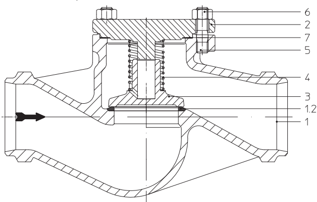
Рис. 4: CHECKO®-V - DG SE PN40 1.0619+N
