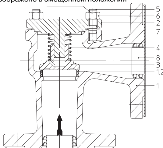
Рис. 2: CHECKO®-V - ECK PN16-40 EN-JS1049 / 1.0619+N
