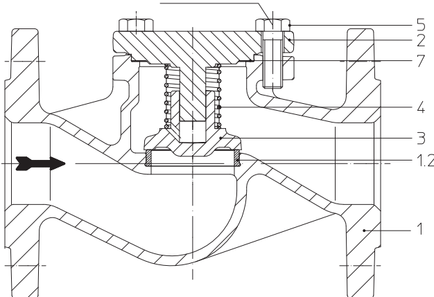
Рис. 3: CHECKO®-V - DG PN6-16 EN-JL1040
