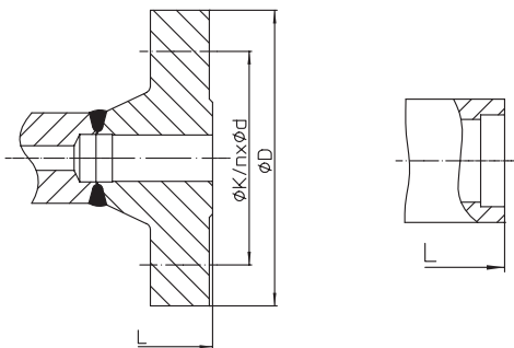
Фиг. 600....1 (PN400) с фланцами
