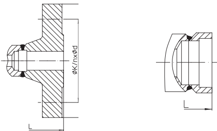
Фиг. 600....1 с фланцами
