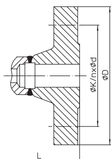
Фиг. 600...1 с фланцами
