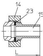
Фиг. 600...5 с резьбовым соединением под приварку
