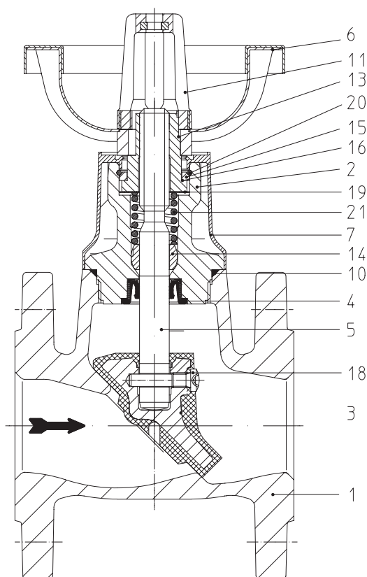
Рис. 1: EURO-WEDI Габаритная длина FTF-14
