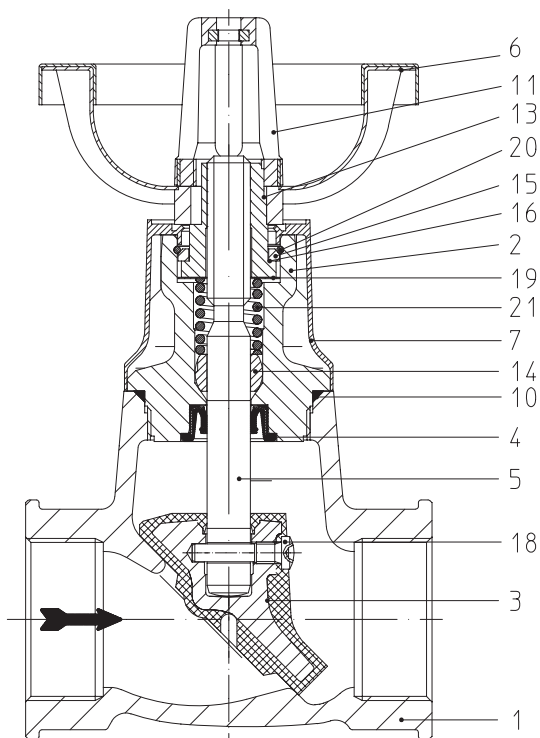
Рис. 1: EURO-WEDI Габаритная длина FTF-14
