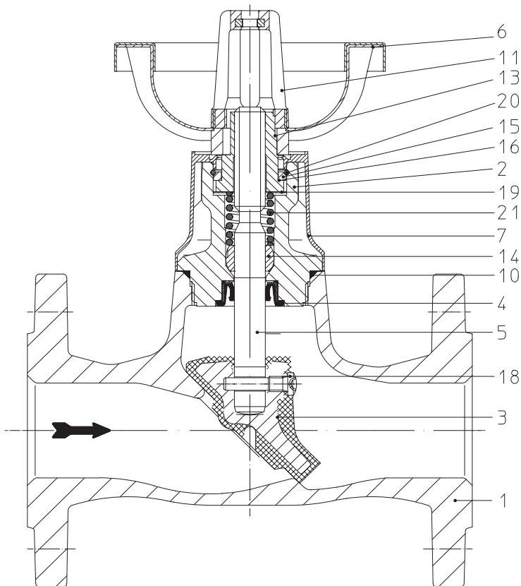
Рис. 4: EURO-WEDI Габаритная длина FTF-1
