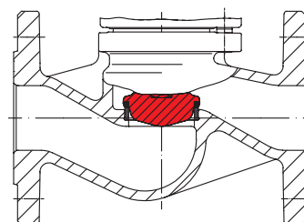
Дроселирующий затвор с мягким уплотнением из PTFE + 25% графита, максимальная рабочая температура 200°C (макс. доп. \Delta P см. Приложение: Характеристики расхода)
