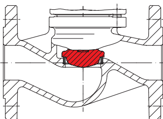
Дроселирующий затвор (макс. доп. \Delta P см. Приложение: Характеристики расхода)
