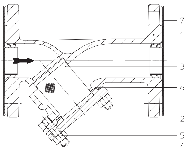
Рис. 3: Грязеуловитель - Y (1.4408)
