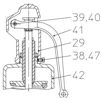
Констр. 902 / 912 / 903 / 904 / 922 / 924 / 945 / 946
