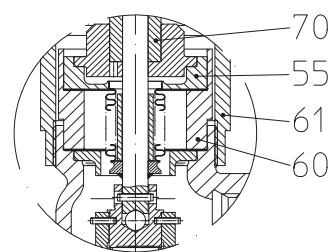
Сильфон- серия 940
