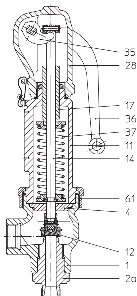
Констр. 941
