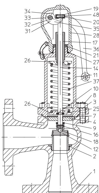
Констр. 921
