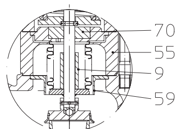
Сильфон
