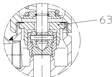
Затвор серия 950
