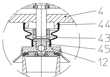
Мягкое уплотнение
