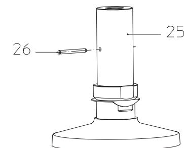
Рис. 15: BR460 DN15-150
