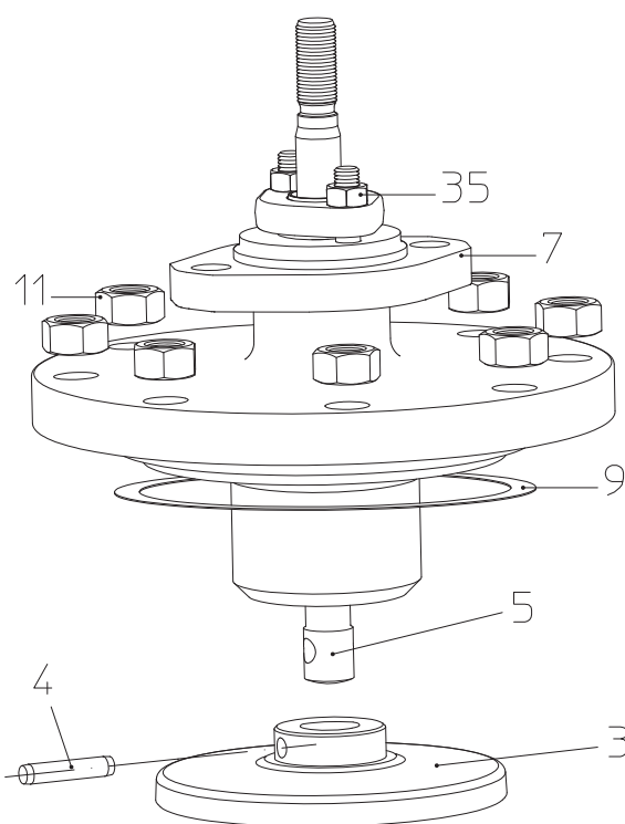
Рис. 18: BR405 DN125-150
