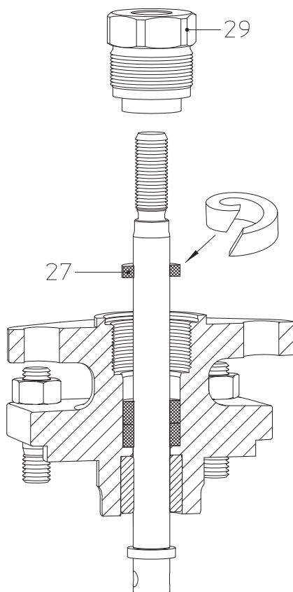
Рис. 11: сальниковая набивка DN15-100 Рис. 12: сальниковая набивка DN125-150
