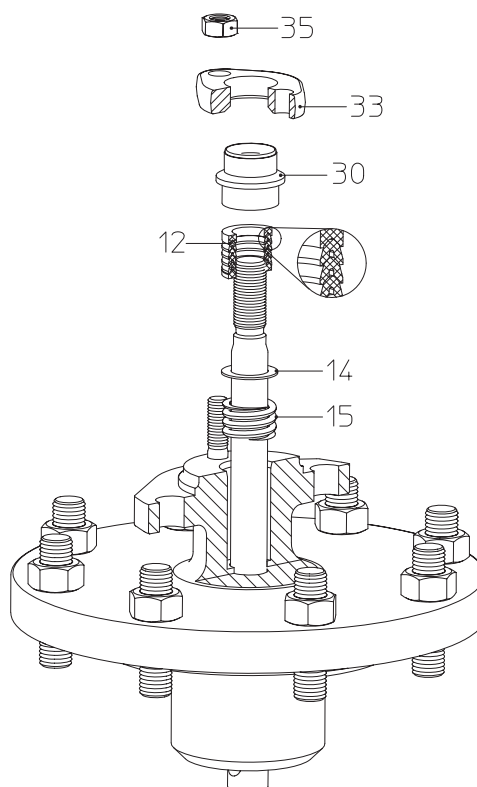
Рис. 9: сальниковые кольца DN15-100 Рис. 10: сальниковые кольца DN125-150
