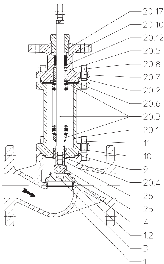
Рис. 2: BR 460 стандартное исполнение
