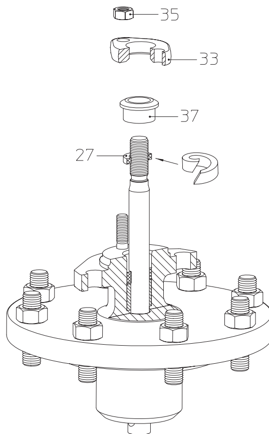
Рис. 11: сальниковая набивка DN15-100 Рис. 12: сальниковая набивка DN125-150
