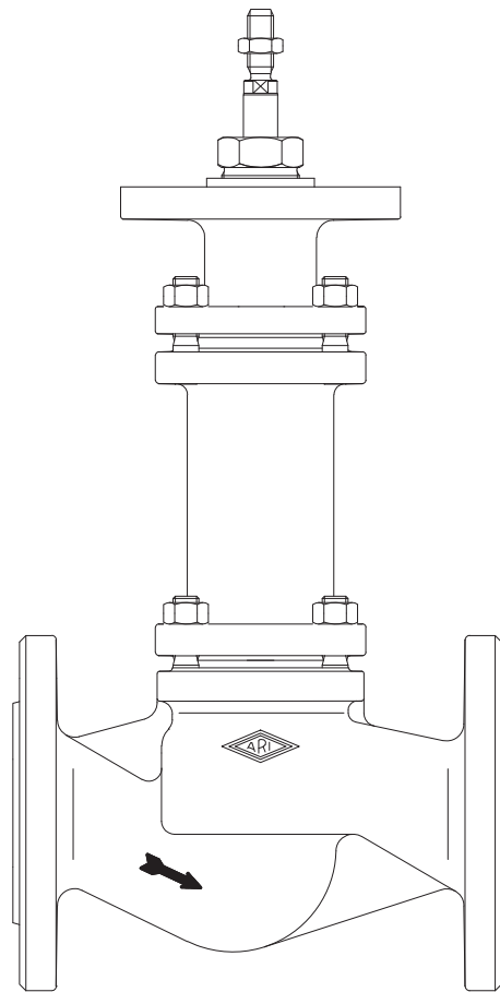
BR 460
