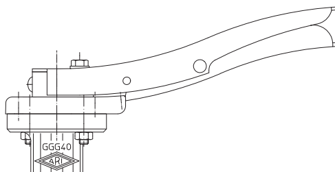
Рис. 3: Стопорный рычаг ZESA® / GESA®
